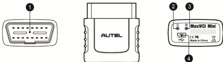
图 2-2 蓝牙诊断接口设备
