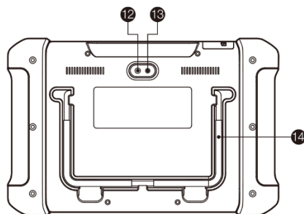
图 2-3 906S 平板诊断设备后视图
