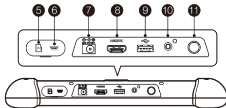
图 2-2 906S 平板诊断设备俯视图
