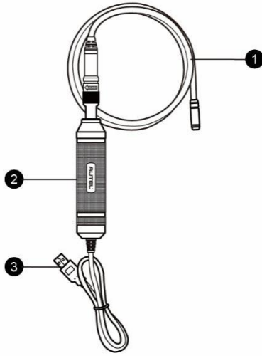
图 16-1 高清内窥镜
